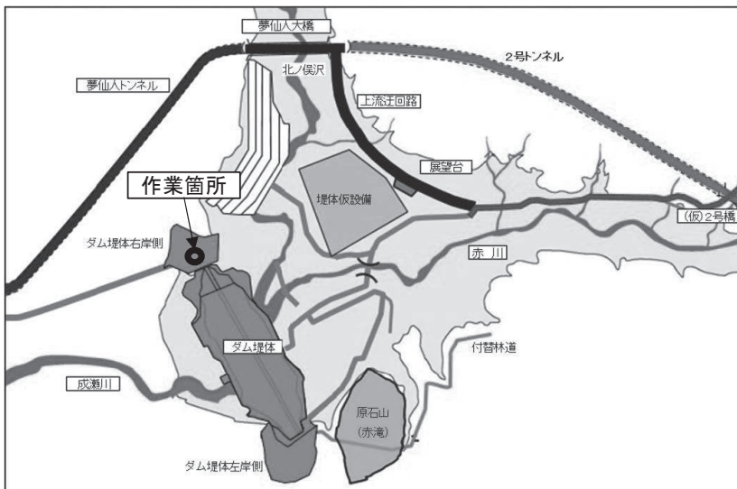
成瀬ダムの平面図
