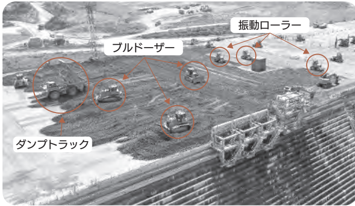
▲無人の建設機械による施工
