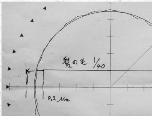
<真円度の測定チャート>真円に対して波線が製品の研削面の凸凹を表す。スケール1目盛りは0.2μメートルまさに0.06の究極のブレである。
