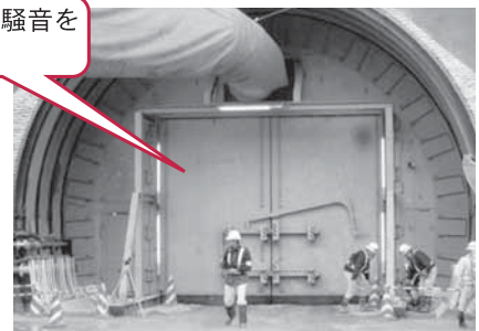
トンネル工事の防音壁設置状況
