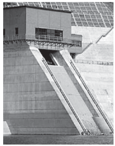
選択取水設備のイメージ (七ヶ宿ダム：宮城県七ヶ宿町)
