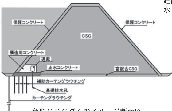
台形CSGダムのイメージ断面図
