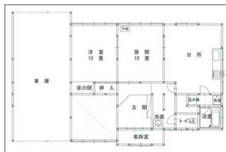
間取り
