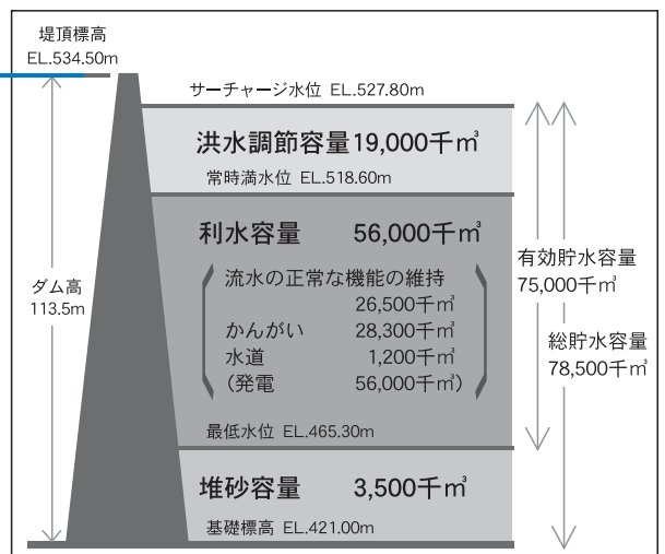
貯水池容量配分図
