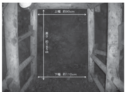
支保工を設置しトンネルを補強した状況
